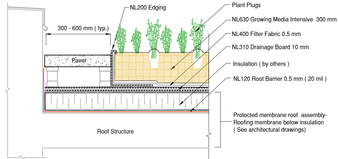
2 Flora Garden Paver Edge Detail
